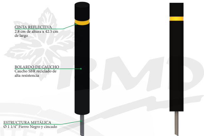
ESTRUCTURA METALICA
