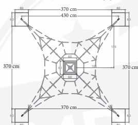
PLANTA - DADOS
