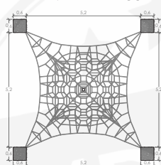
PLANTA - DADOS
