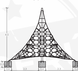
CORTE
